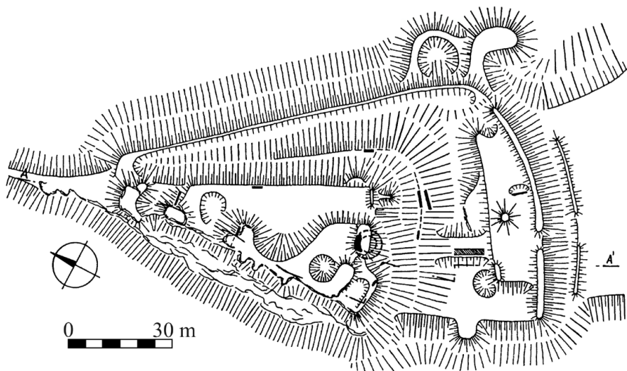
Obr. 2. Hrad Hluboký. Půdorys hradu. Reprofoto: Plaček, M.: Ilustrovaná encyklopedie moravských hradů, hrádků a tvrzí. Praha 2001, obr. 406.
