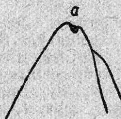
DUDINCE a - mrtvý kráter
