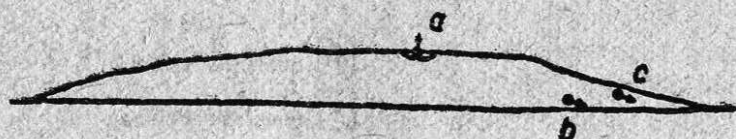
TRI SLIAČE /kupa Certovica/ a - velký kráter b - malý kráter c - pramen
