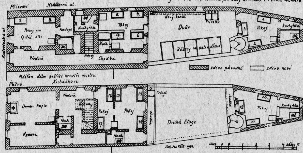
Obr. 9. Dům v Kateřinské ulici (nyní U tržnice) číslo 8. Plán na úpravu domu pro účely špitálu z roku 1778.
