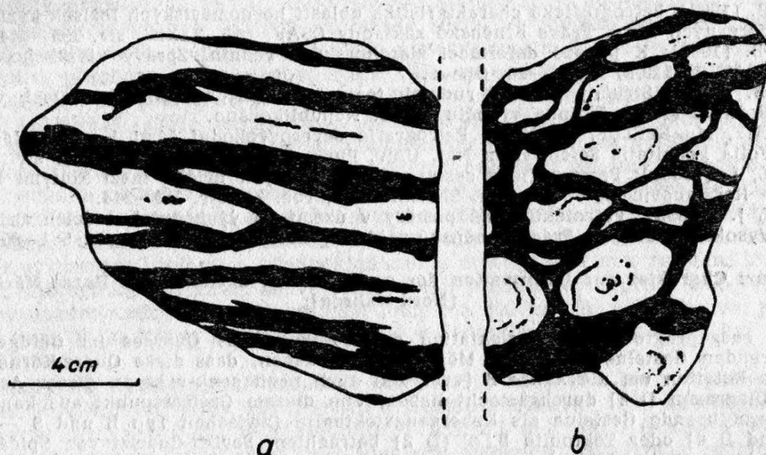
Obr. 3: Rudní agregáty s hlušinou (černě) v přeměněném keratofyrovém popelovém tufu; a — rovnoběžně s lineací, b — kolmo k lineaci. Nová jáma, III. patro.
