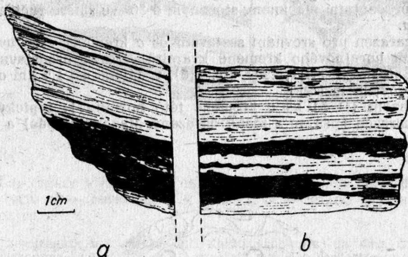
Obr. 1: Sericitická břidlice s proužky pyritu a hlušiny (černě). a — rovnoběžně s lineací, b — kolmo k lineací. Jáma Jaromír, I. patro.
