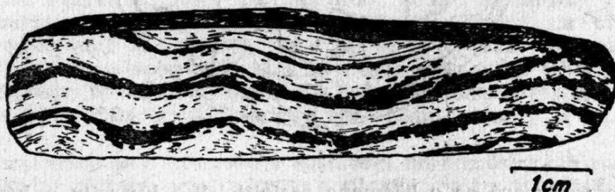
Obr. 2: Páskovaná břidlice se zvrásněnými vrstvičkami rud a hlušiny (černě); kolmo k ose B'. Jáma Jaromír, III. patro.
