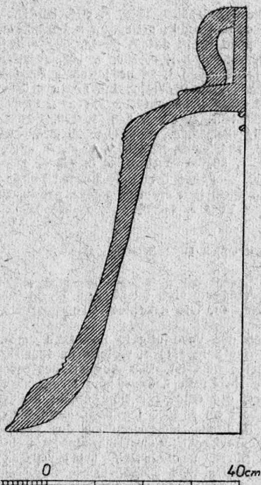
1. Žebro zvonu Zachariáše Milnera z r. 1603 (Podbřežice, okr. Vyškov). Kreslil V. Burian
