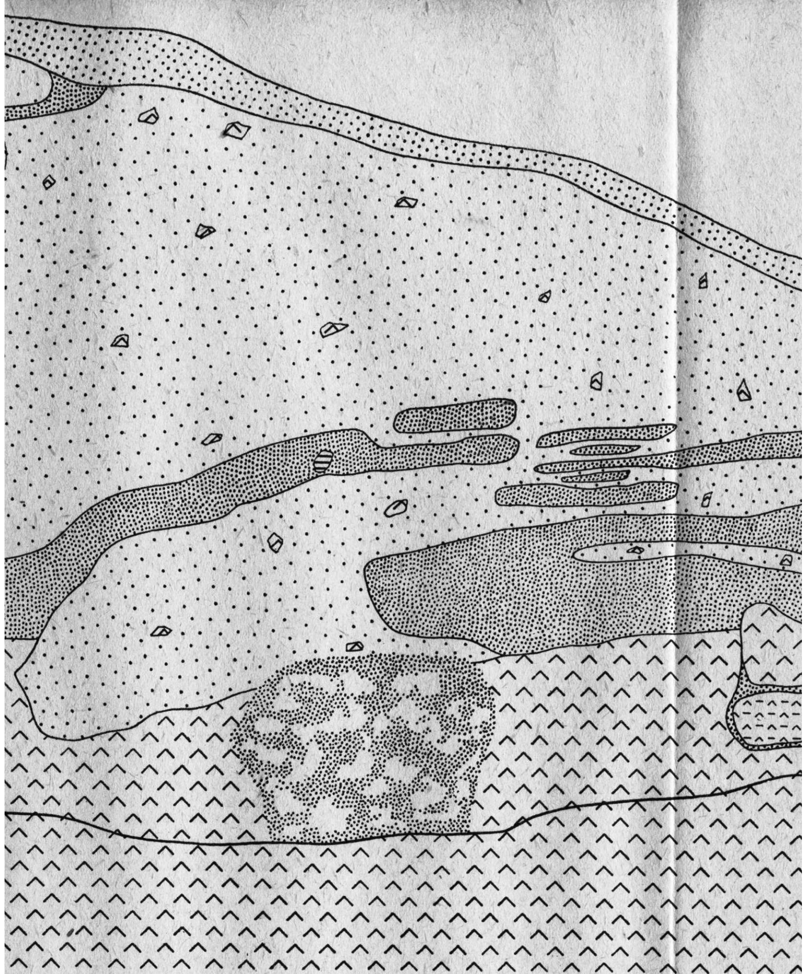
Obr. 2. Profilový řez vnitřním valem na hradisku Podborský, J. Štelcl 1966, kreslil J. 1 — okatá rula, 2 — plagioklasová rula, rula ( p > Kž ), 4 — granát-biotit-muskovitice na s uhlíky, 7 — porušená hlína s uhlíky uhlíků, 9 — písčité polohy, 10 — humus.
