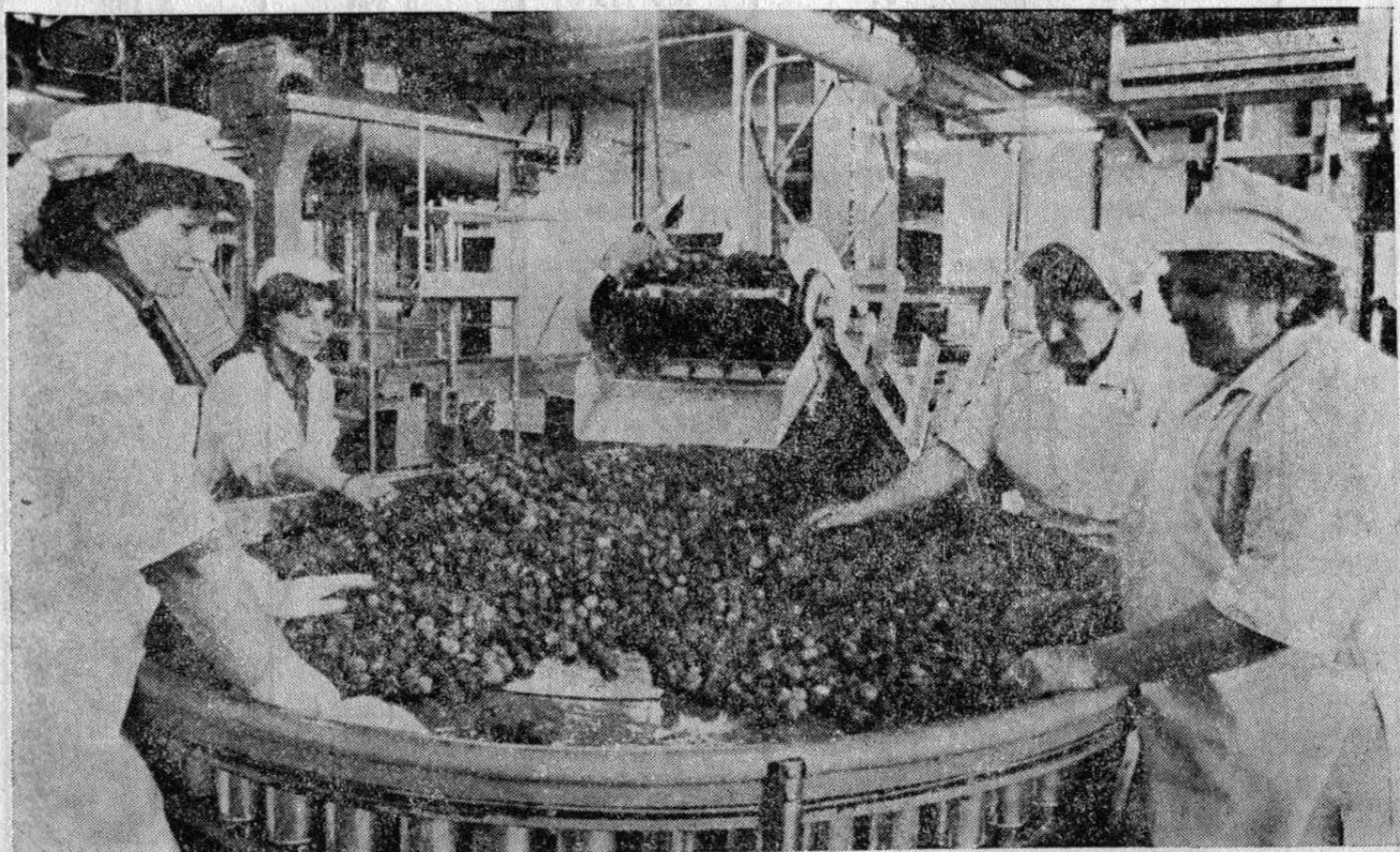
Rekonstruovaná linka – plnicí stůl (zpracování jahod, 1981), foto archiv Seliko
