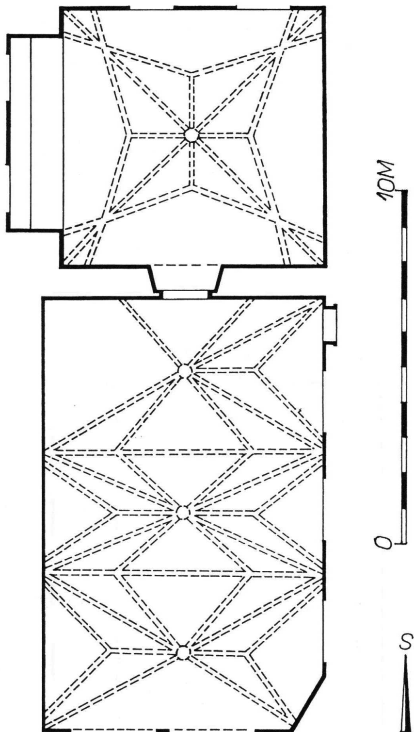
2. Půdorys kleneb místností v prvním patře. Kresba a zaměření Z. Otruba, 1998.
