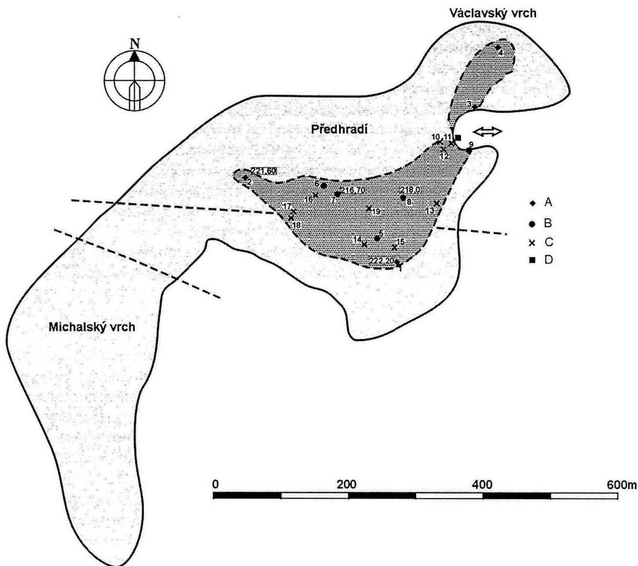
Obr. 2: Rozšíření plioleistocenních písků v oblasti petrské a václavské (dómské) kry.
