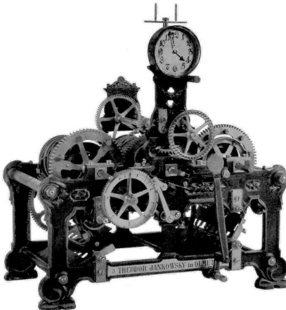
Stroj věžních hodin, výrobce L. Hainz, Praha, dodavatel T. Jankowsky, Olomouc, 1902 (Foto: P. Rozsival)
