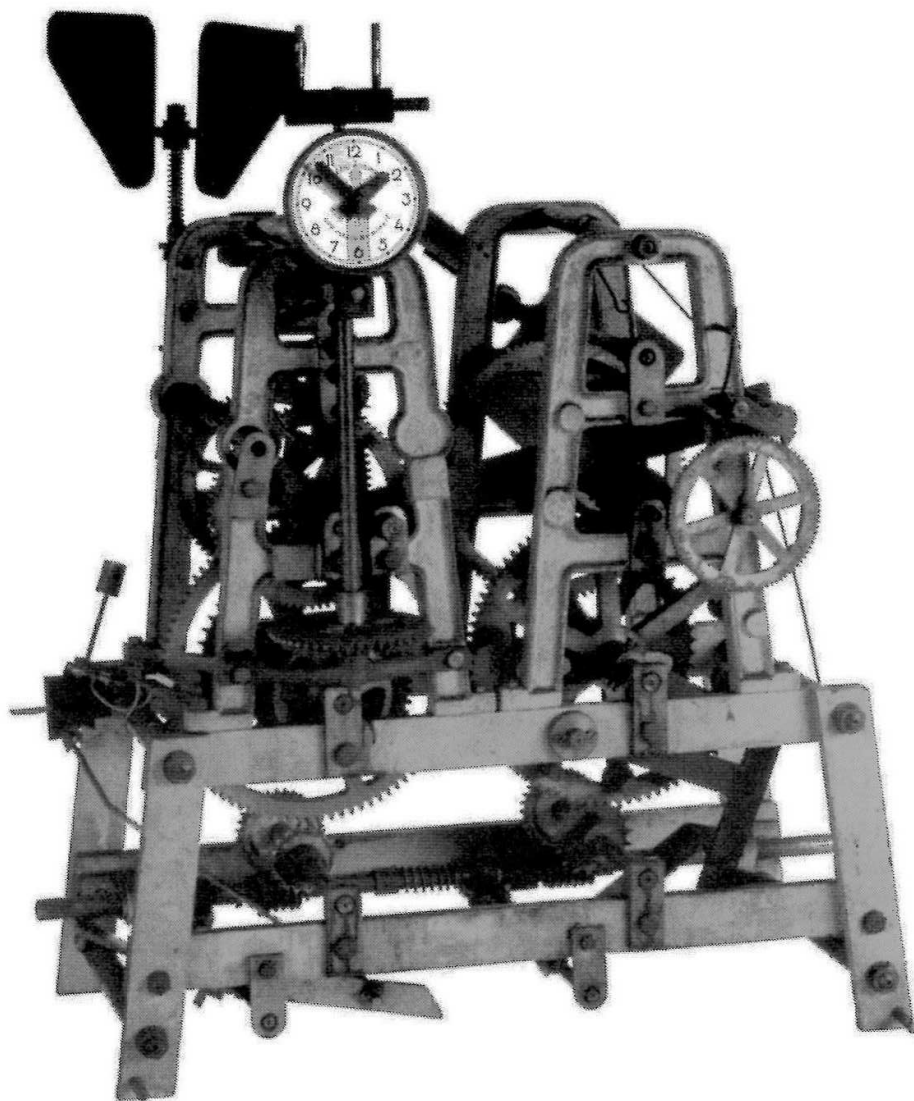
Věžní hodinový stroj z Nové radnice v Ostravě, OPP Vyškov, 70. léta 20. století (Foto: P. Rozsívál)
