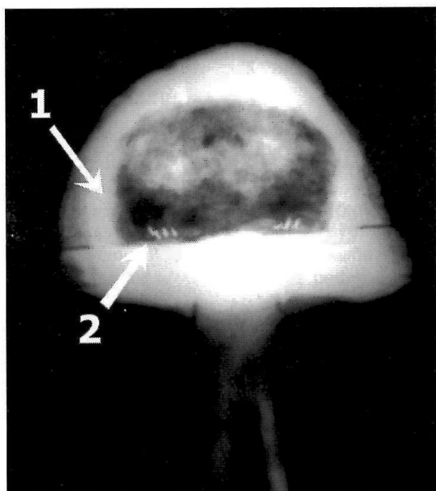
Rentgenový snímek fragmentu čepele: 1 – nýt spojující korunu hlavice s její základnou, 2 – zbytky stříbrných tautů (Vojenská nemocnice Hradisko)
