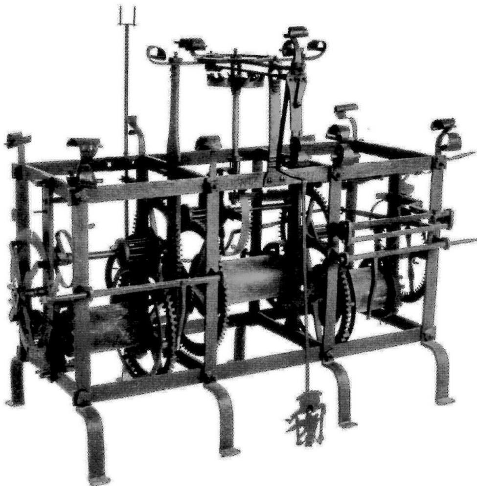
Stroj věžních hodin, F. Lang, Uherské Hradiště, 1734 (Foto: P. Rozsival)
