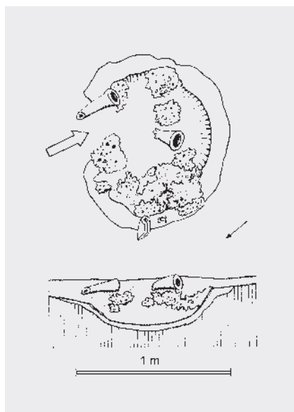
Obr. 6. Žerotín. Kresba odkrytého pyrotechnického zařízení č. I. Repro: Pruš, J. (ed.): Dějiny hutnictví železa v Československu 1. Praha 1984, s. 53, obr. 9.
