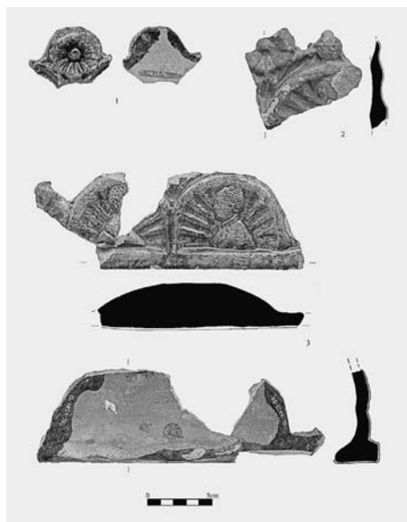
Obr. 5. Olomouc. Zeleně glazované kamnové nástavce z Horního náměstí č. o. 25 (1, 3) a Dolního náměstí č. o. 40 (2). Foto: Pavel Rozsívál a Lukáš Hlubek, kresba: Lukáš Hlubek.
