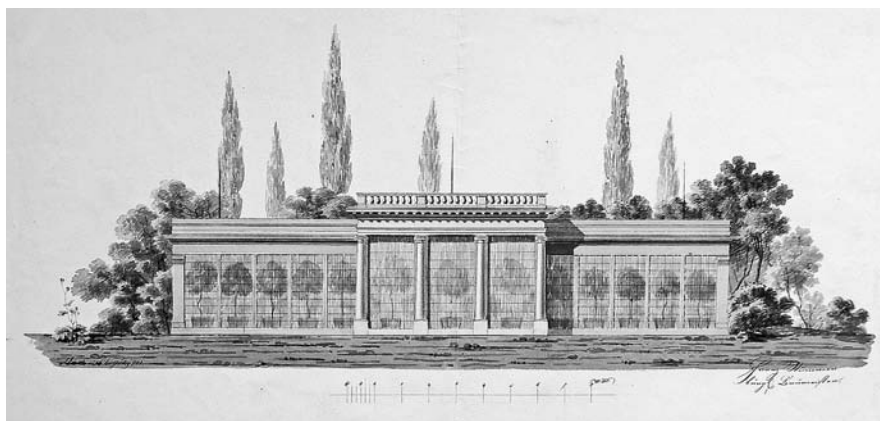
Obr. 6. Franz Stummer, Fasáda oranžerie pro 40 kusů stromů, 1831, Muzeum a galerie v Prostějově, inv. č. 015336. Foto: Ondřej Belšík.
