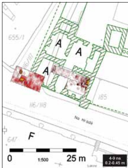
Obr. 3. Zbytky věžice v jihozápadním nároží budovy bývalého fojstství, zjištěné geofyzikální prospekci na podkladu plánu bývalého fojstství na Michalském návrší ze 17. století. Plán podle V. Nešpora, prospekce podle M. Moníka. Digitalizace: J. Grégr, Národní památkový ústav, územní odborné pracoviště v Olomouci.
