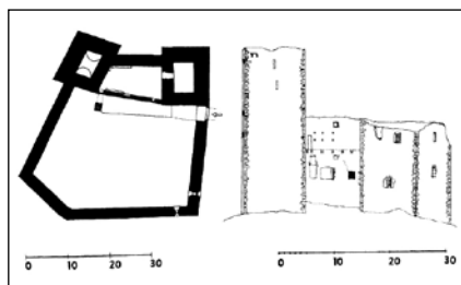
Obr. 8. Románské jádro hradu Landštejna (podle D. Menclové).
